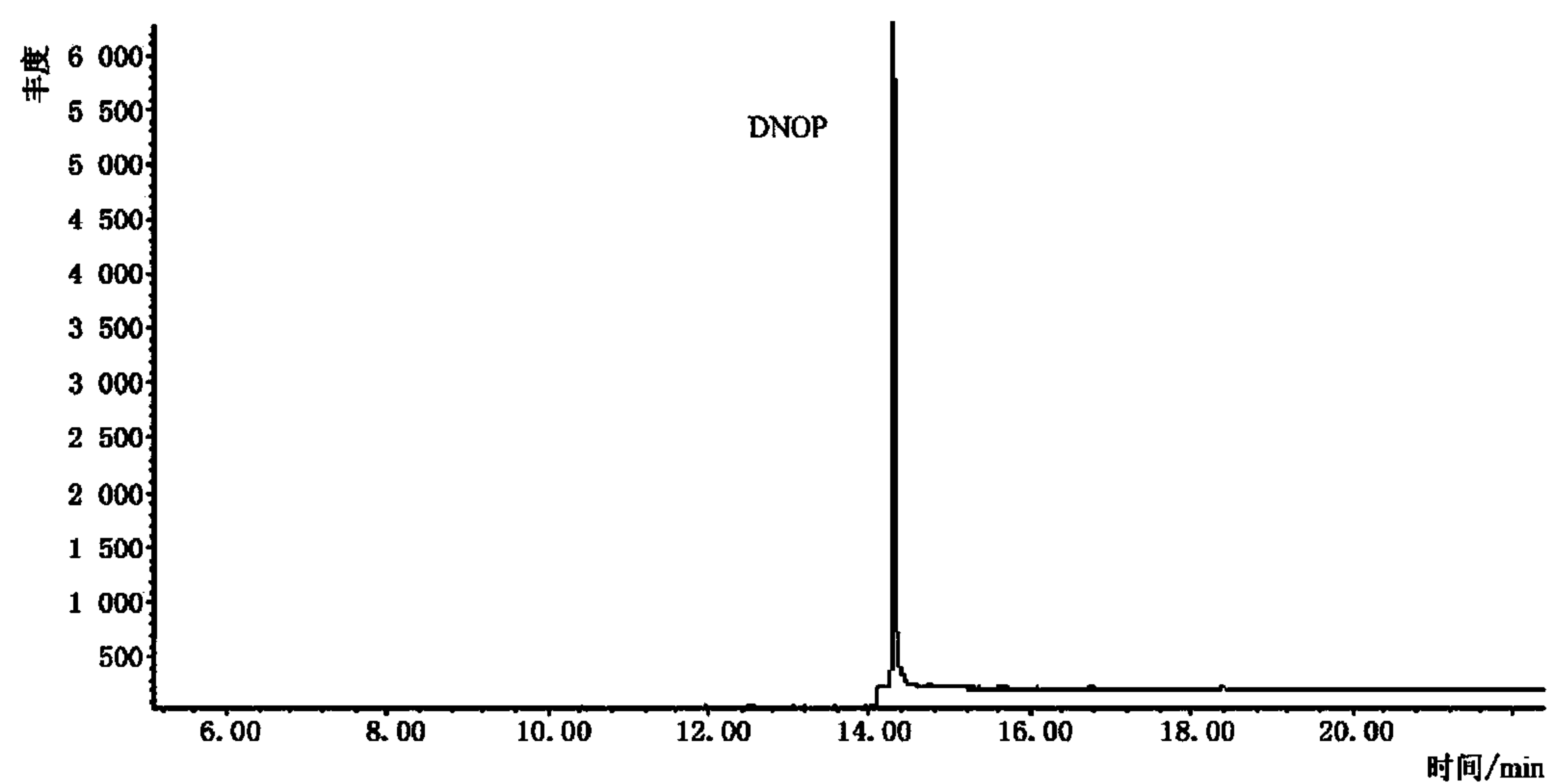
图 C.3 DNOP 的 GC-MS 选择离子色谱图(SIM)
