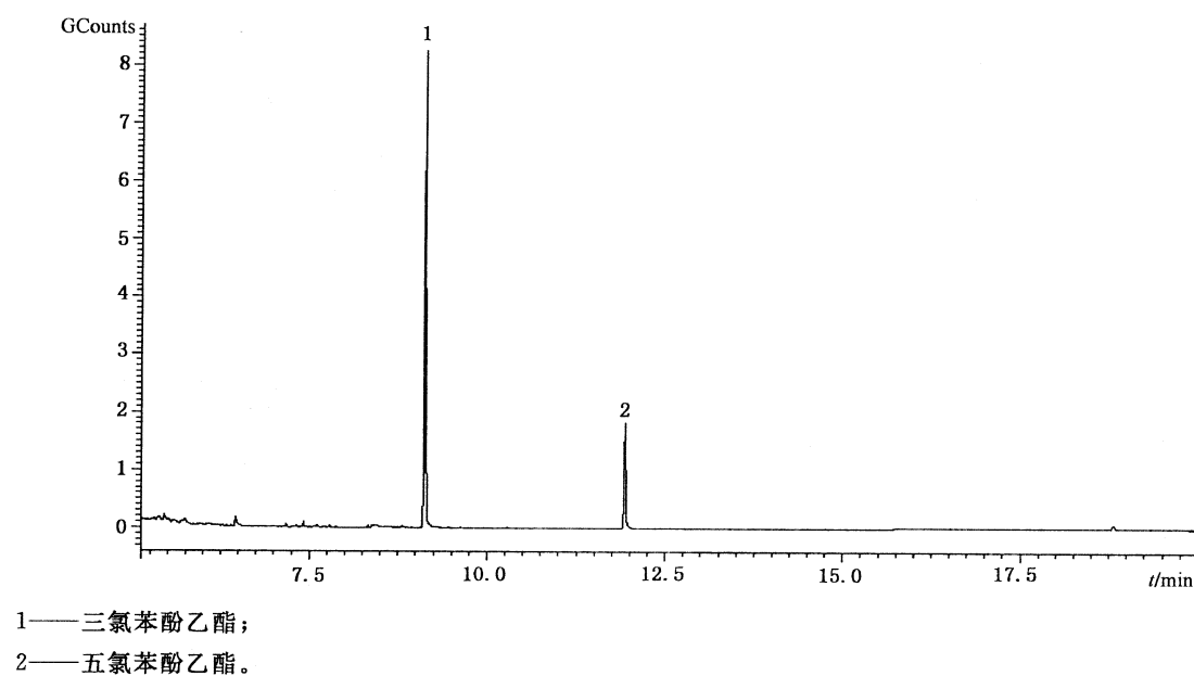
图 D.1 五氯苯酚及内标物衍生物的典型气相色谱-质谱图
